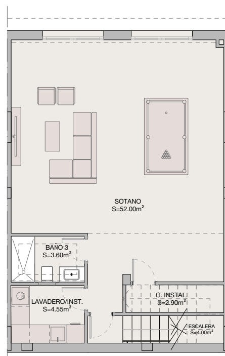
planta sotano
