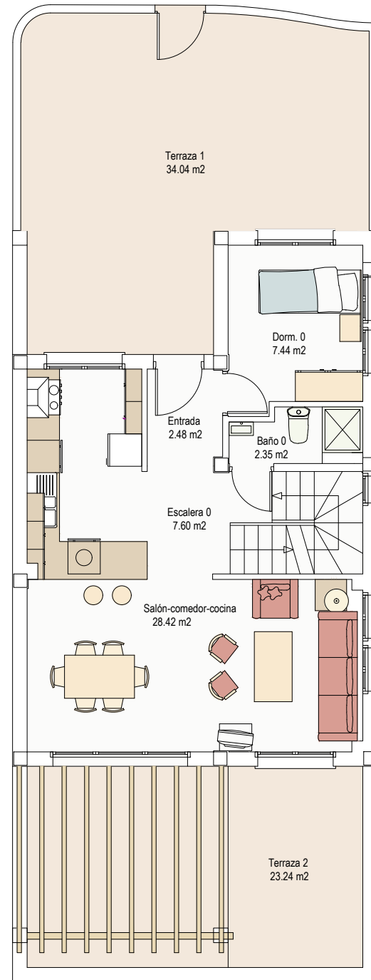
Planta baja
