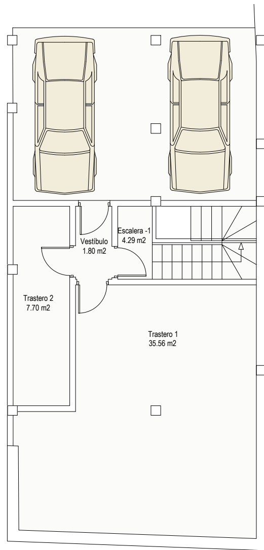
Planta sótano
