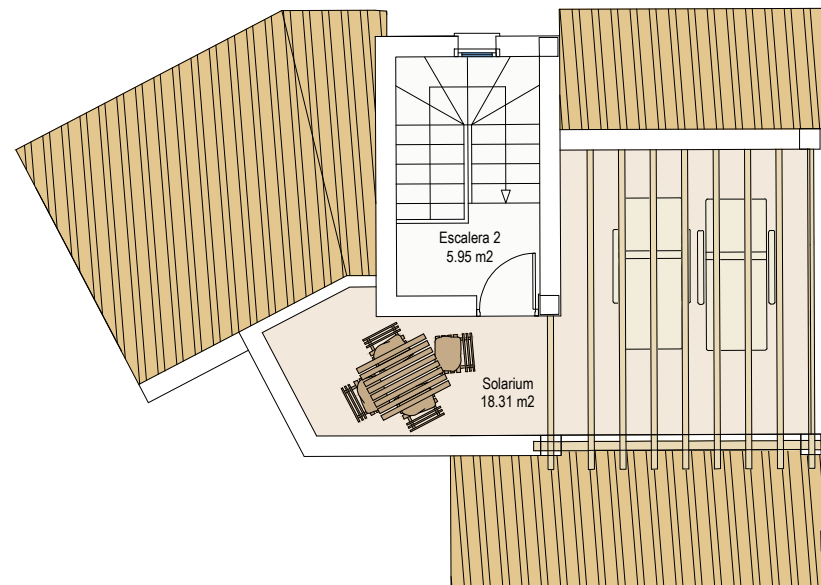
Planta cubierta
