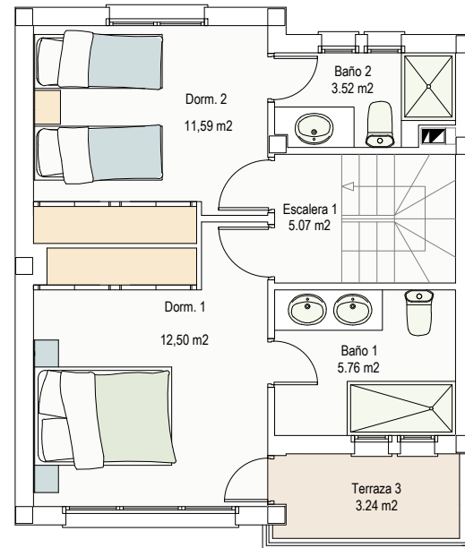
Planta primera
