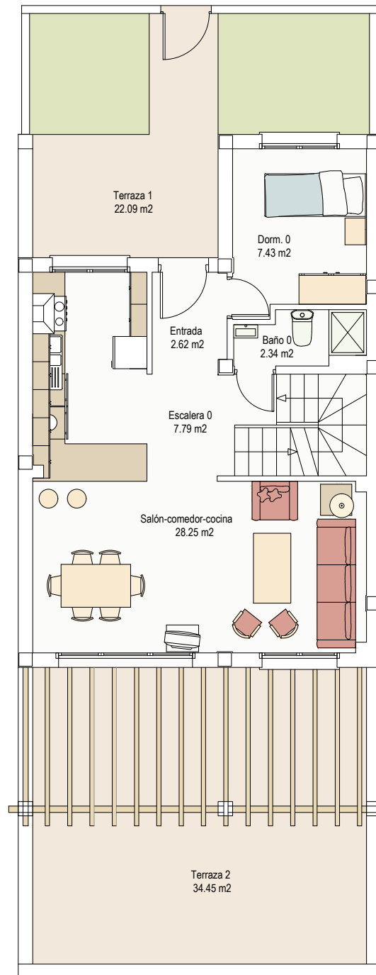
Planta baja
